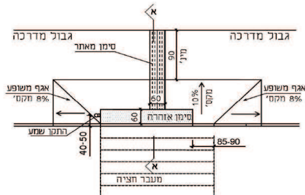
12א - מבט על
