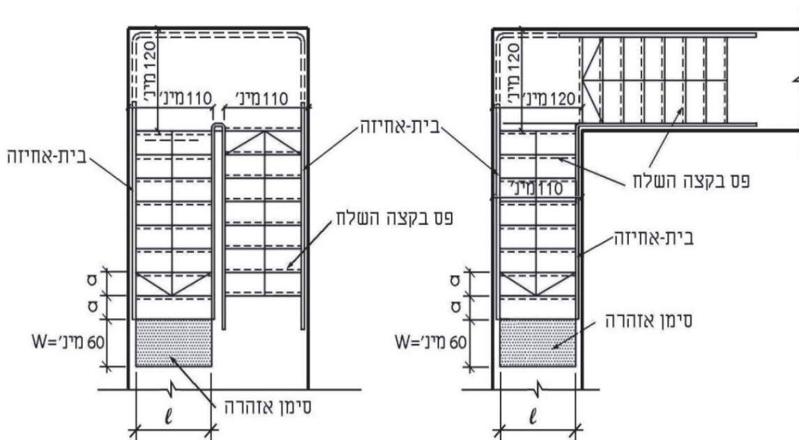
12ב - מדרגות פרסה
