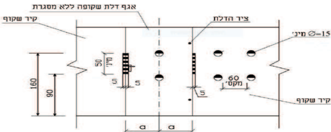
12 ג - סימון דלת שקופה משולבת בקיר שקוף
