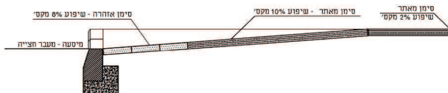
12ב - חתך א-א
